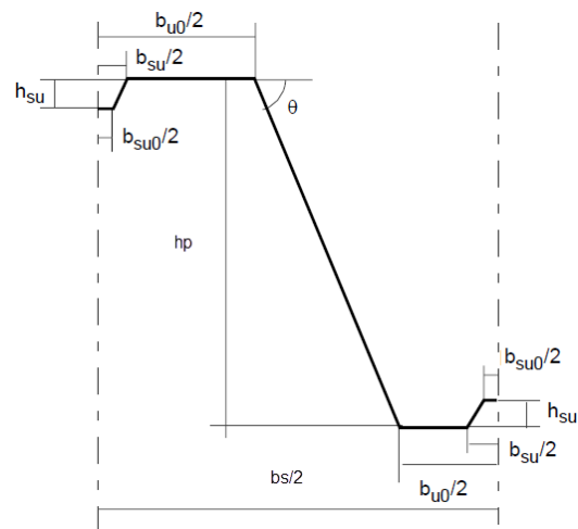
Διαστάσεις χαλυβδόφυλλου τραπεζοειδούς και μορφής υποσκαφής
