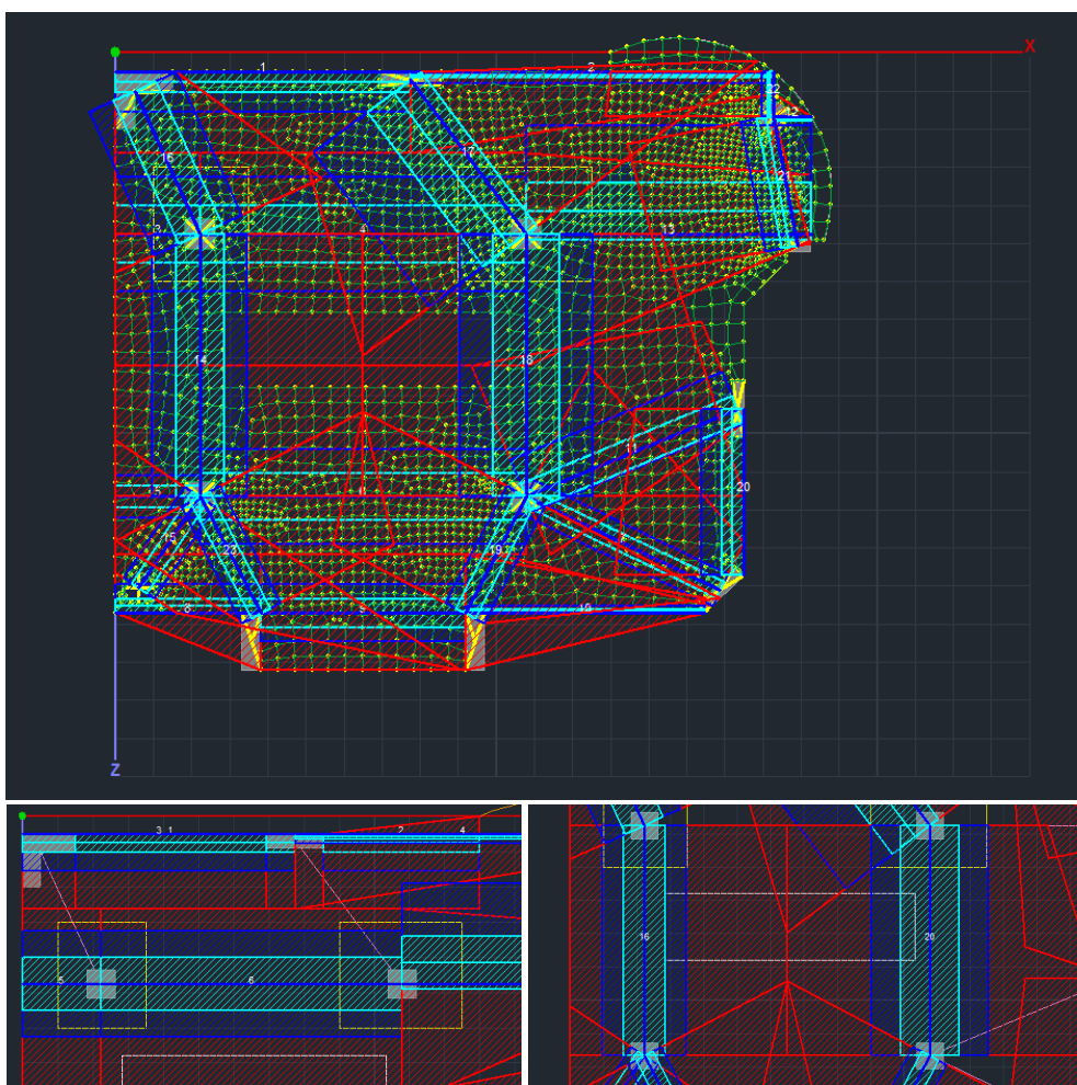
Λωρίδες Φορτίσεων κατά μήκος του άξονα X και Z
