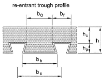
Διαστάσεις χαλυβδόφυλλου τραπεζοειδούς και μορφής υποσκαφής
