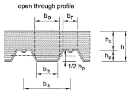
Διαστάσεις χαλυβδόφυλλου τραπεζοειδούς και μορφής υποσκαφής
