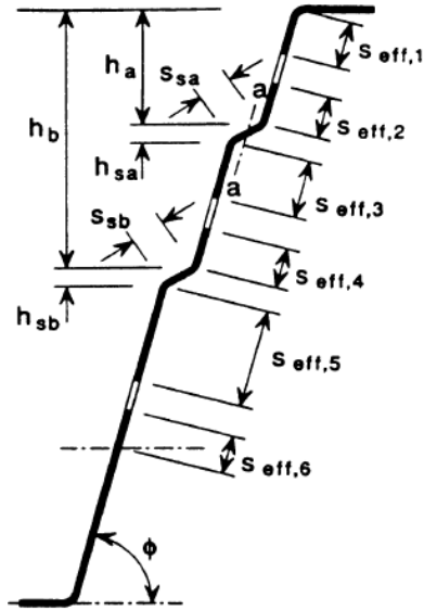
Διαστάσεις ενισχύσεων κορμού
