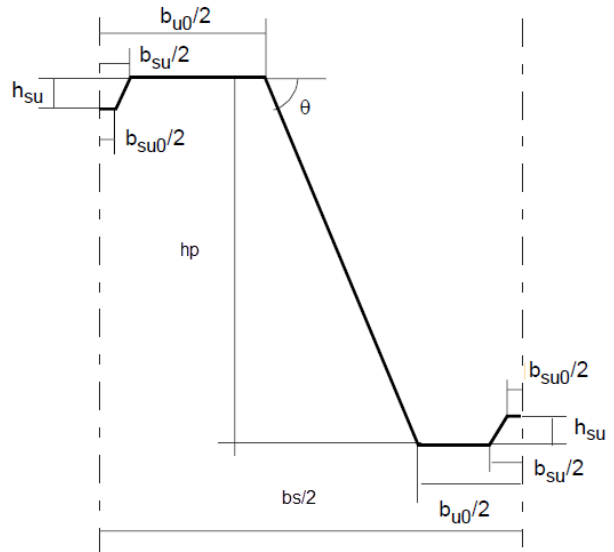
Διαστάσεις ενισχύσεων πέλματος
